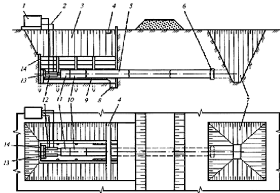
1 - насосная станция; 2 - газопровод; 3 - рабочий котлован; 4 - водоотводной лоток; 5 - защитный футляр; 6 - лобовая обделка (нож); 7 - приемный котлован; 8 - приямок для сварки защитного футляра; 9 - направляющая рама; 10 - нажимной патрубков; 11 - нажимная заглушка; 12 - гидродомкраты; 13 - башмак; 14 - упорная стенка
