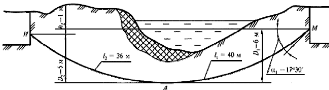
Рисунок Л.4 - Расчетные параметры пилотной скважины
