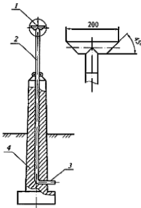
1 - оголовок; 2 - вытяжная труба; 3 - отводная труба; 4 - фундамент
