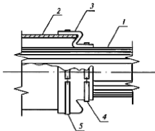
1 - трубная плетть; 2 - защитный футляр; 3 - резиновая манжета; 4 - малый хомут; 5 - большой хомут
