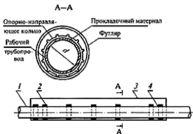
1 - газопровод; 2 - опорно-направляющее кольцо; 3 - футляр; 4 - прокладочный материал
